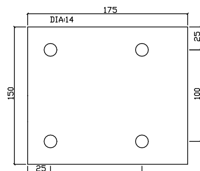
CLF4 (SCALE 1:7)
