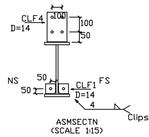
ASMSCTN (SCALE 1:15)
