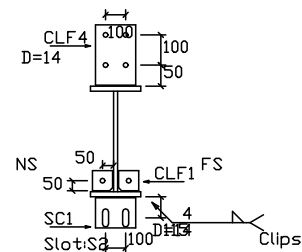
ASMSECTN (SCALE 1:15)
