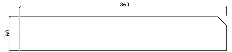
ST4 (SCALE 1:7)
