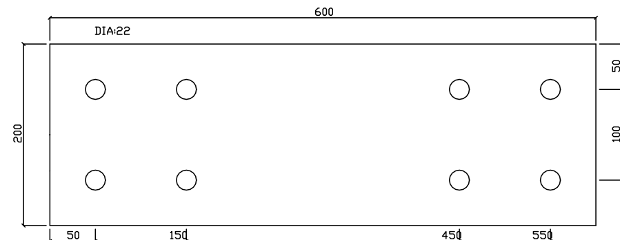
EP2 (SCALE 1:5)
