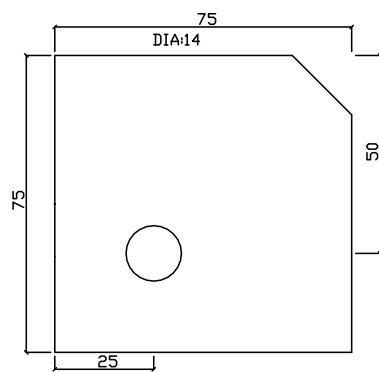
CLF1 (SCALE 1:15)
