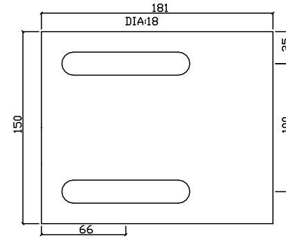
SC1 (SCALE 1:7)
