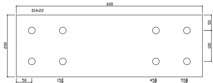
EP2 (SCALE 1:5)
