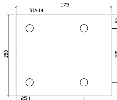
CLF4 (SCALE 1:7)
