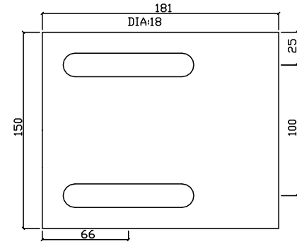
SC1 (SCALE 1:7)
