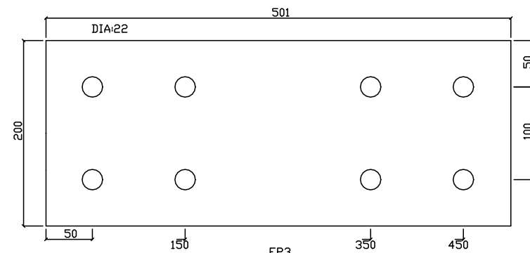
EP3 (SCALE 1:5)
