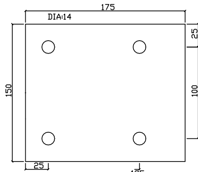
CLF4 (SCALE 1:7)
